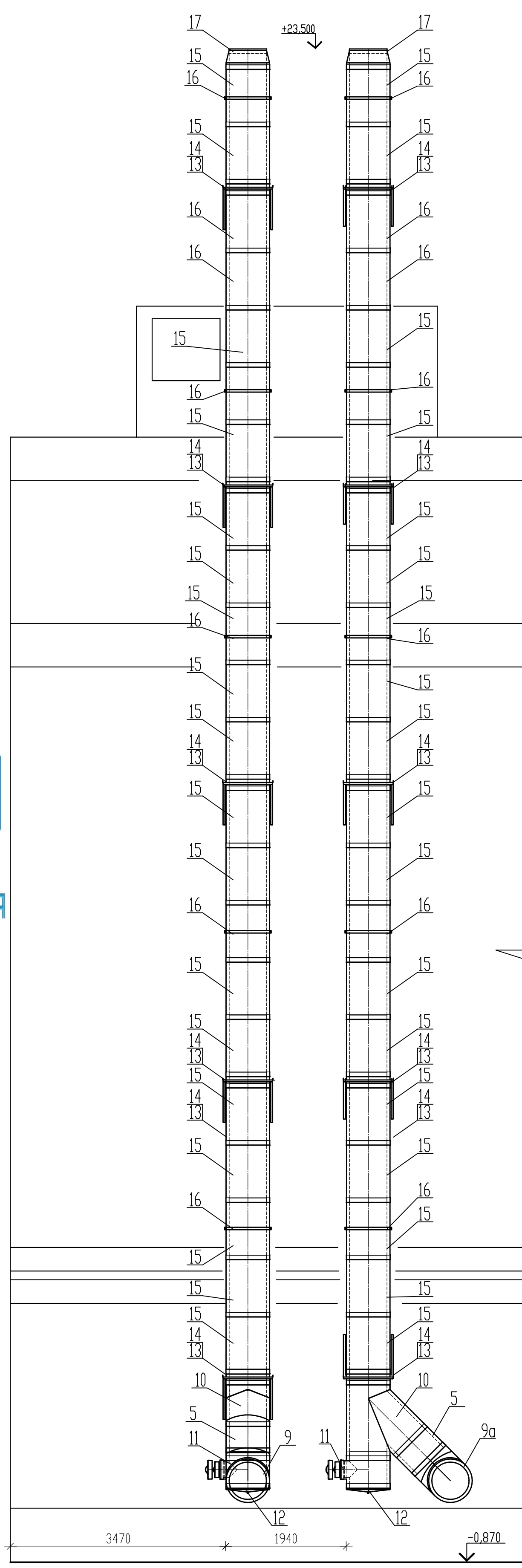
Разрез 2-2
