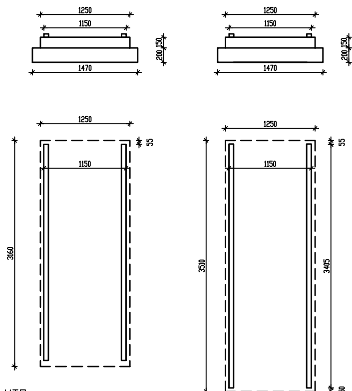
Раскладка демпферных подушек
