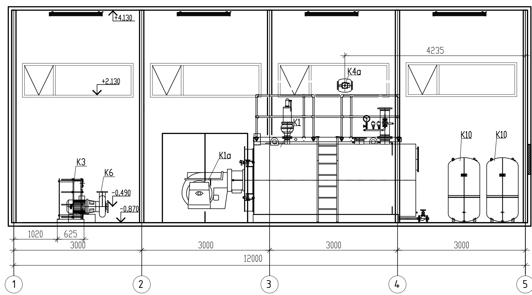
Разрез 1-1
